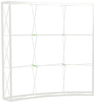
STRUCTURE SEULEMENT
